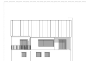
Ansicht Nord Bestand 1:200
